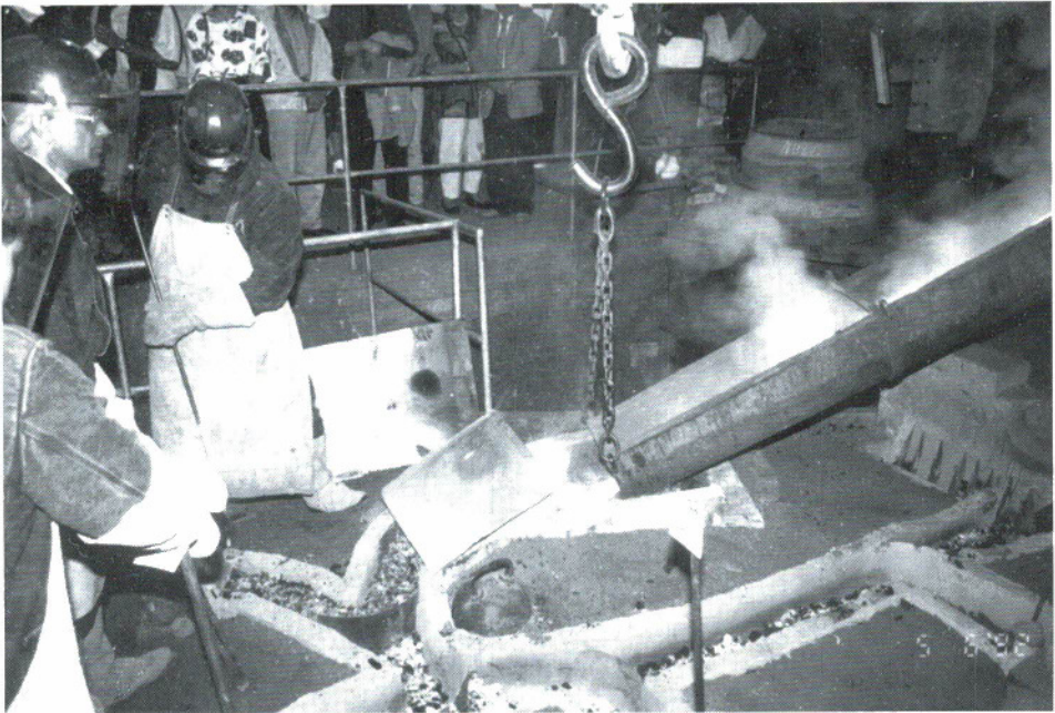
Unser Bild zeigt den Glockenguß der Elsener Glocke
